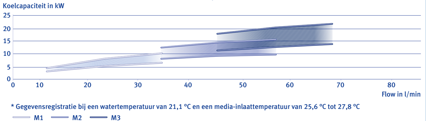
Overzicht van de vermogens ThermoGenius™ Water M1 – M3* Koelcapaciteit
